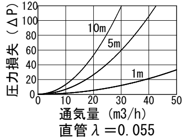
抵抗損失曲線 φ50 標準
