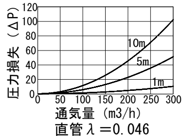
抵抗損失曲線 φ125 標準
