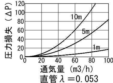
抵抗損失曲線 φ75 標準
