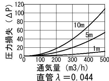
抵抗損失曲線 φ150 標準
