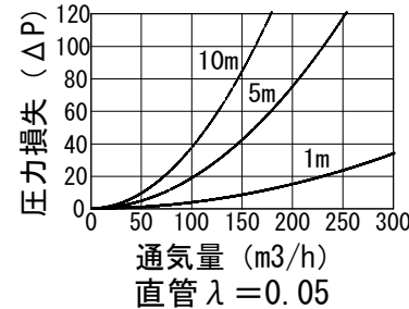
抵抗損失曲線 φ100 標準
