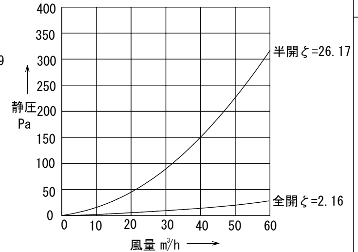
圧力損失曲線(吹出)
