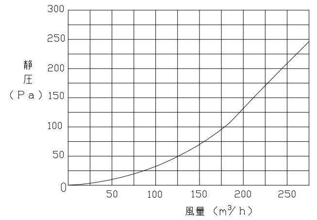
圧損特性
