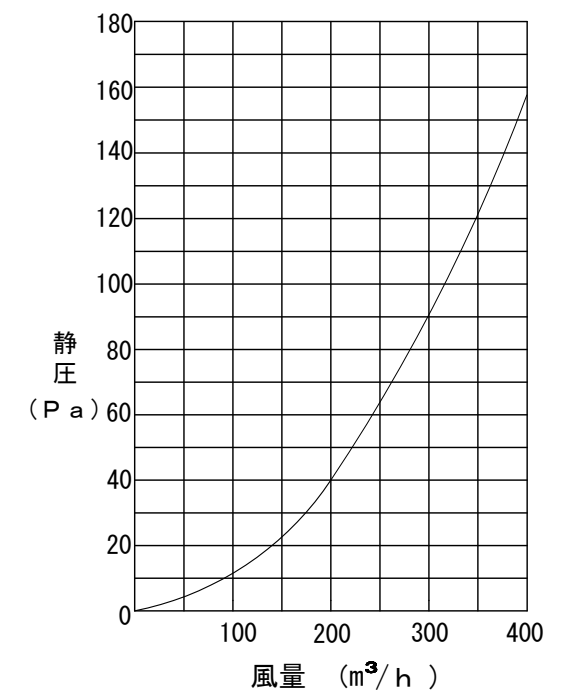
圧損特性
