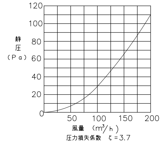
圧損特性
