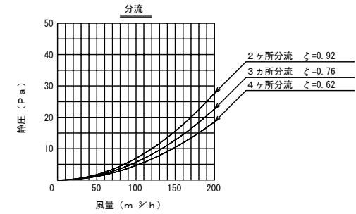
圧力損失曲線
